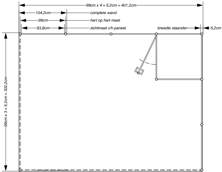
BOVEN AANZICHT
